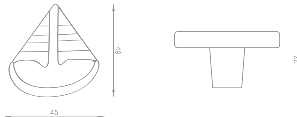
Dimensiones (mm)
